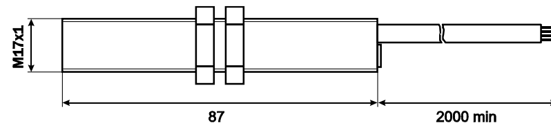
Рис.1. Габаритные размеры фотодатчика МикРА Ф3
